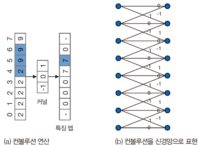
그림 6-9 컨볼루션층의 부분 연결성과 가중치 공유
